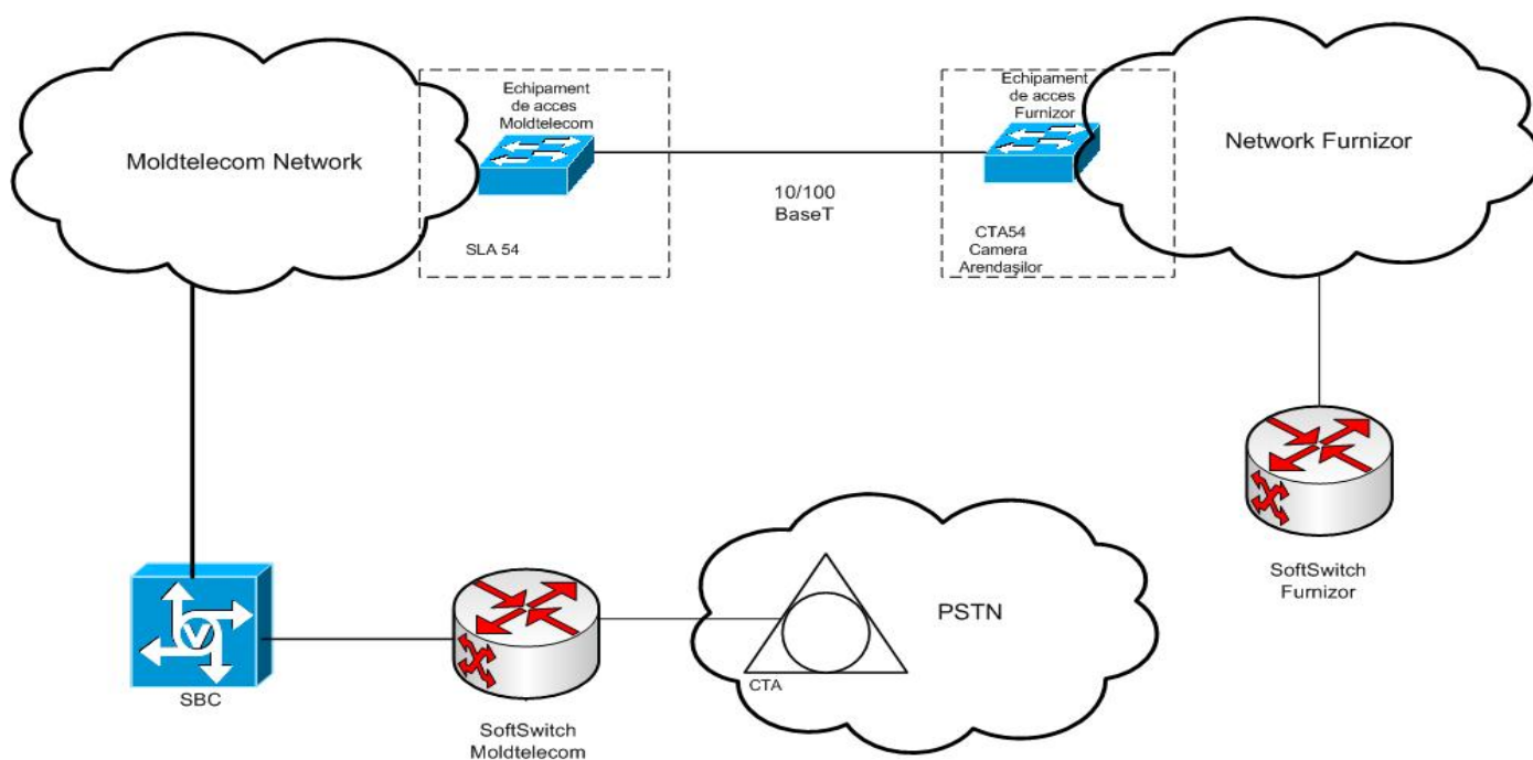
Schema de interconectare MTC – Furnizor prin protocolul SIP-I
